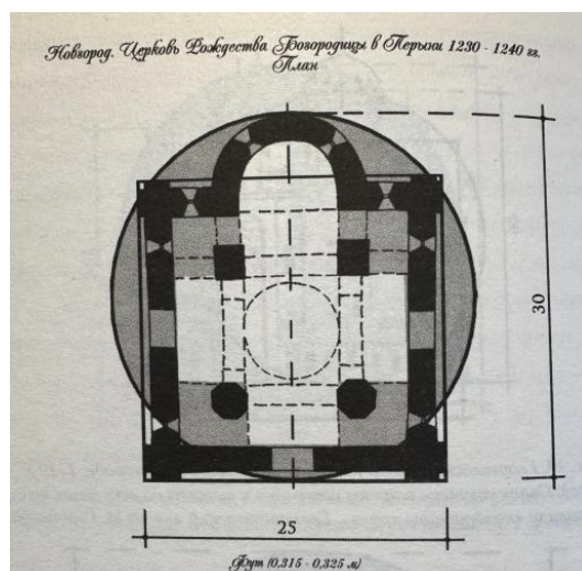
Рисунок 6. Церковь Рождества Богородицы в Перыньском скиту (1230–1240). Новгород. Пример построения плана церкви по правилу «квадратуры круга». Геометрический анализ М. Городовой (источник: [26])
