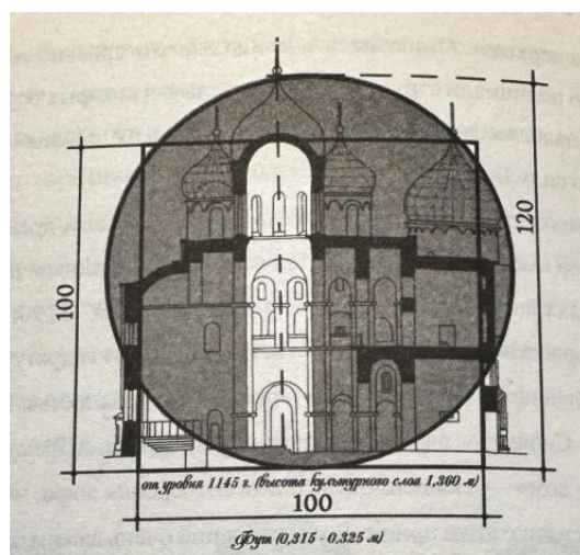
Рисунок 5. София Новгородская. Пример построения высот собора по правилу «квадратуры круга» (источник: [26])
